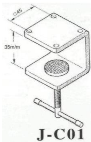
Чертеж струбцины J-C01
