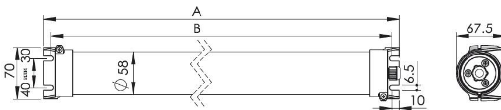
Чертеж светильника (с креплением GS-115)
