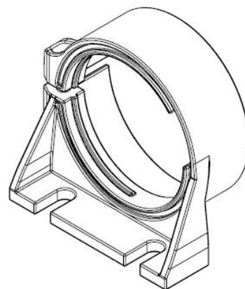
Крепление GS-115
