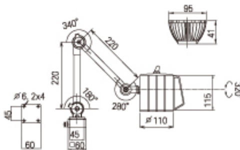
Чертеж светильника LED-M70
