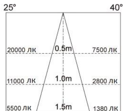
Распределение светового потока
